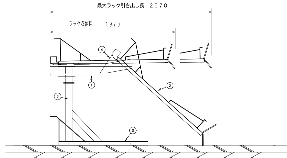
ラック詳細図 S=1/30
